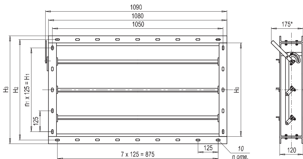
ГАБАРИТНЫЕ РАЗМЕРЫ КВУ-Р
